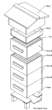
Warre Hive
